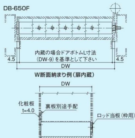
DB-650F納まり例(戸先側からのみメンテナンス可能)
