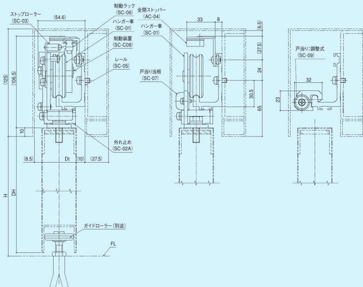
戸先側縦断面
