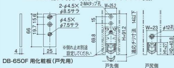
DB-650F H断面推奨切欠(扉内蔵)
