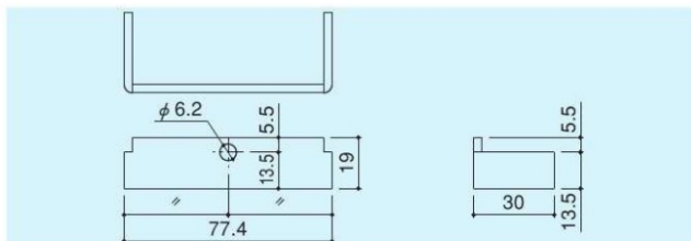
上吊引戸ストッパー
