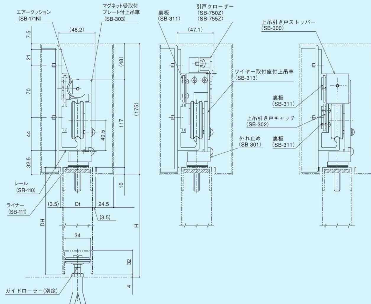
閉止時戸尻側
