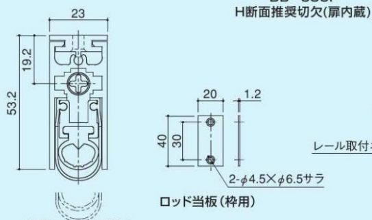
DB-650F H断面推奨切欠(扉内蔵)
