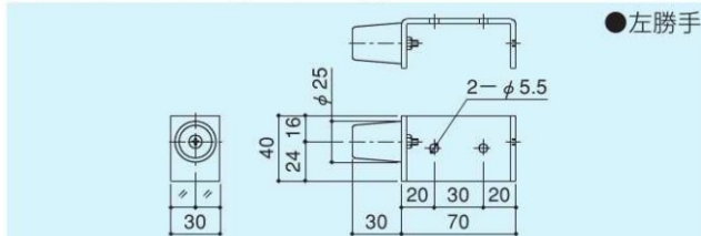
引戸クローザー
