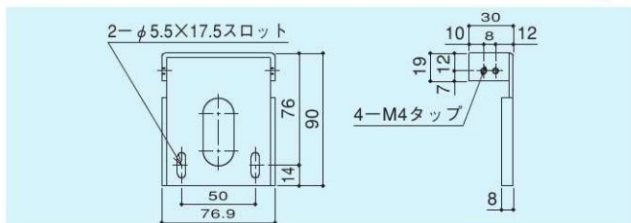
外れ止め
