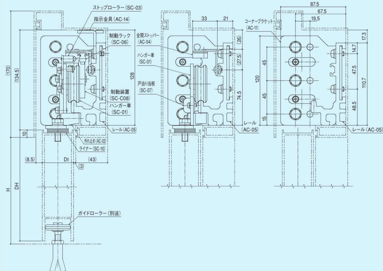
戸先側縦断面
