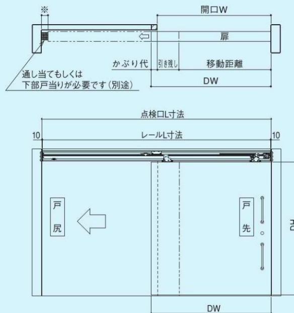
図は左引き(左勝手)です
