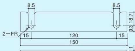
上吊引戸キャッチ
