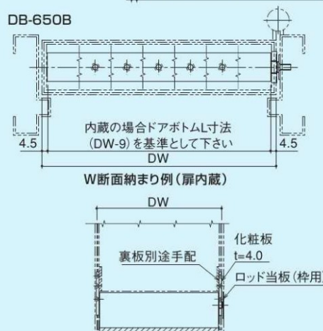
DB-650B納まり例(戸尻側からのみメンテナンス可能)
